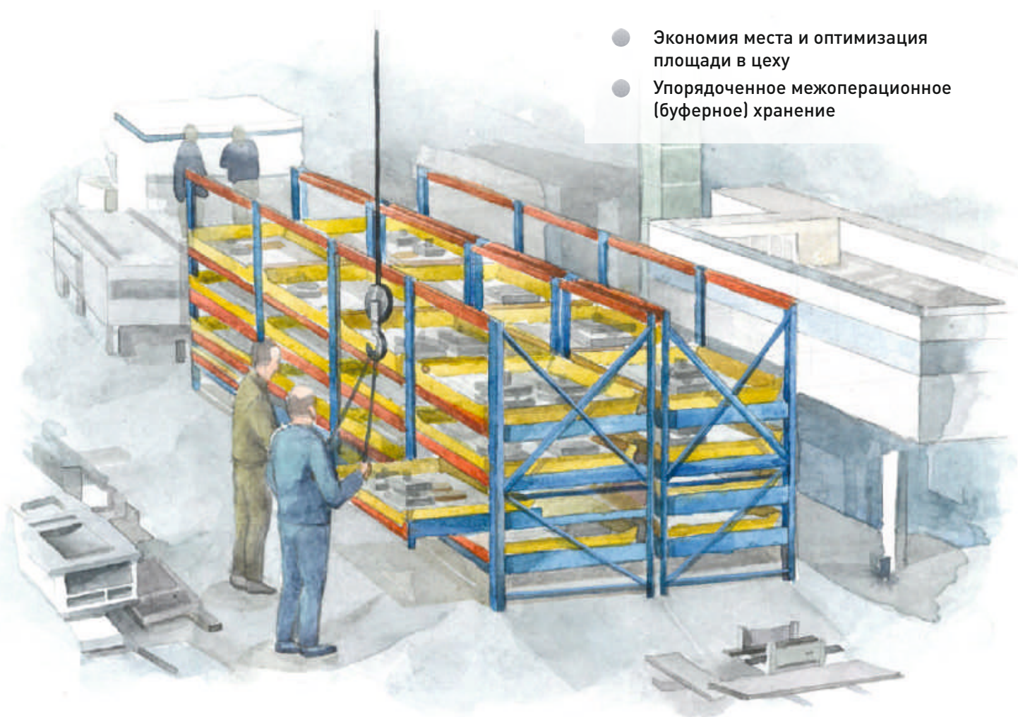
Буферное хранение изделий на стеллаже в цеху
